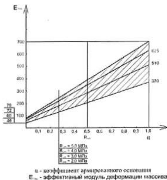
Рисунок Ф.1 - График зависимости эффективного модуля
