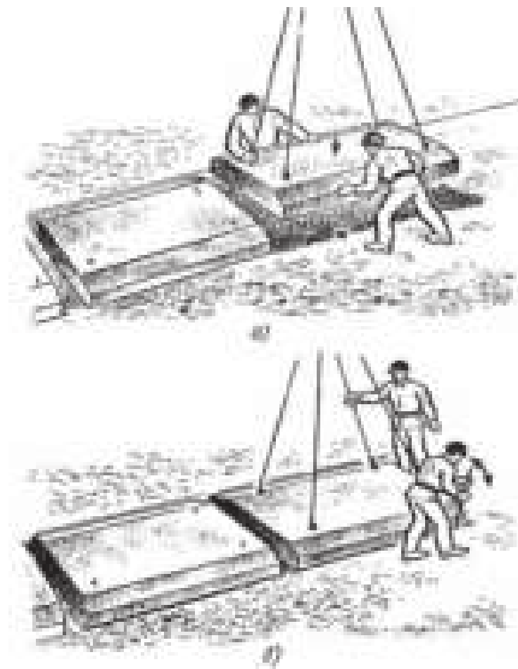
а) опускание на основание; б) выверка положения
