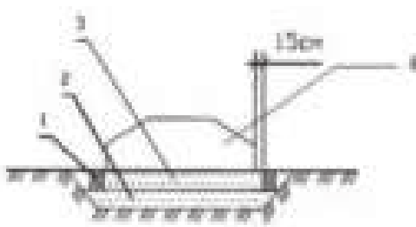
1 – маячные рейки; 2 и 3 – соответственно нижний и верхний слой подсыпки; 4 – фундаментная подушка
